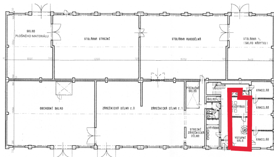
PŮDORYS 2.P. SKUTEČNÉ PROVEDENÍ STAVBY mřížko 1:200
