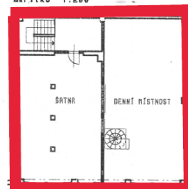
PŮDORYS 2.P. SKUTEČNÉ PROVEDENÍ STAVBY mřížko 1:200
